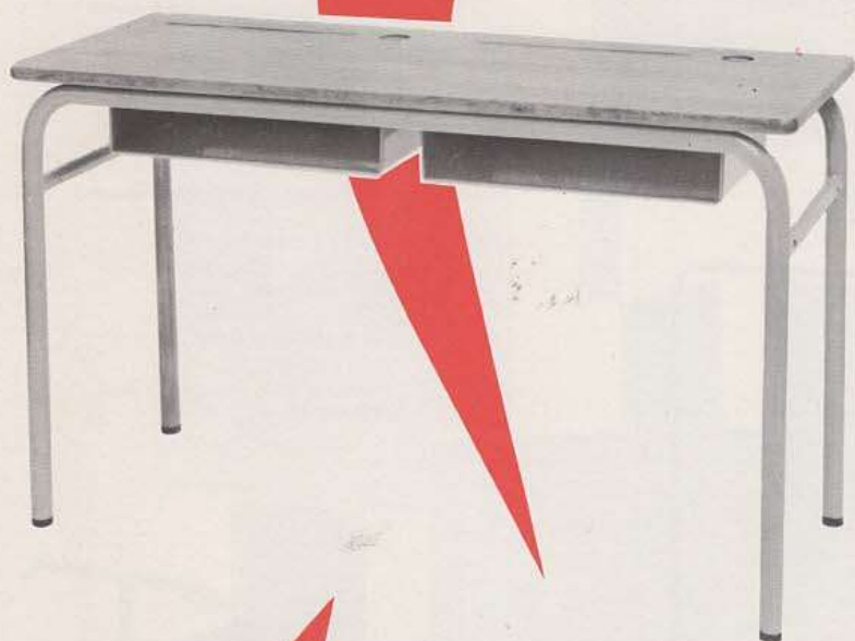
RÉF. 1074 E TABLE DOUBLE A SIÈGES INDÉPENDANTS DÉMONTABLE Ossature tubes émaillés au four de diam. 32 mm Dessus lamellé hêtre verni de 21 mm d'épaisseur Avec ou sans casier porte-livres empilable.
